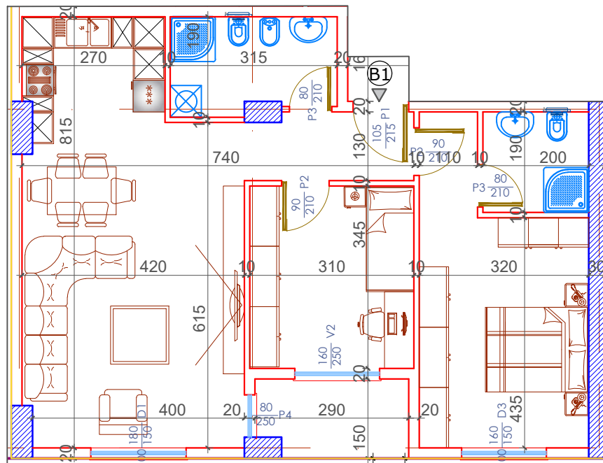
PLANIMETRIA E APARTAMENTIT NR 1 KATI TIP (KATI PARË +5.04) SEKSIONI B SH.1:100
