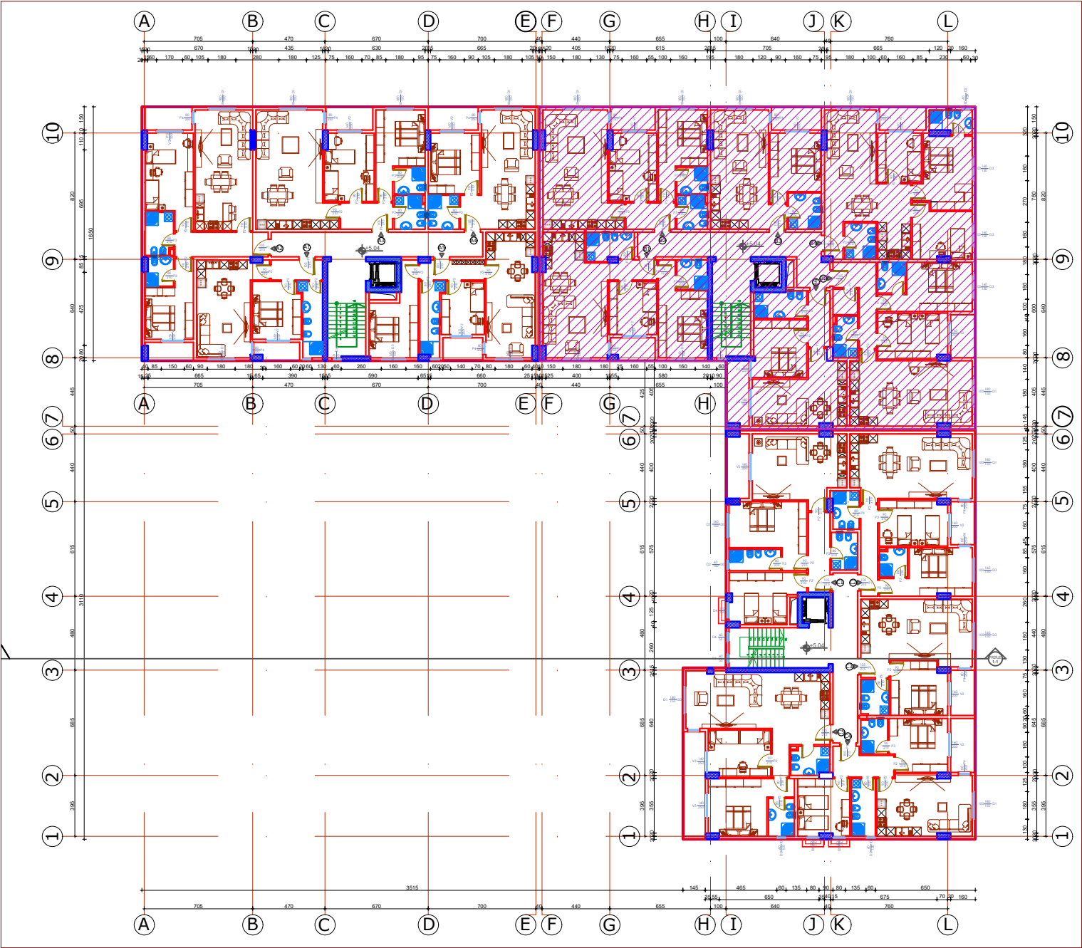
PLANIMETRIA E KATIT TIP (KATI PARË +5.04) , SEKSIONI A SH 1:350
