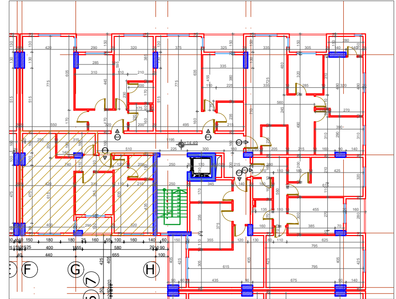
KATI KATËRT
