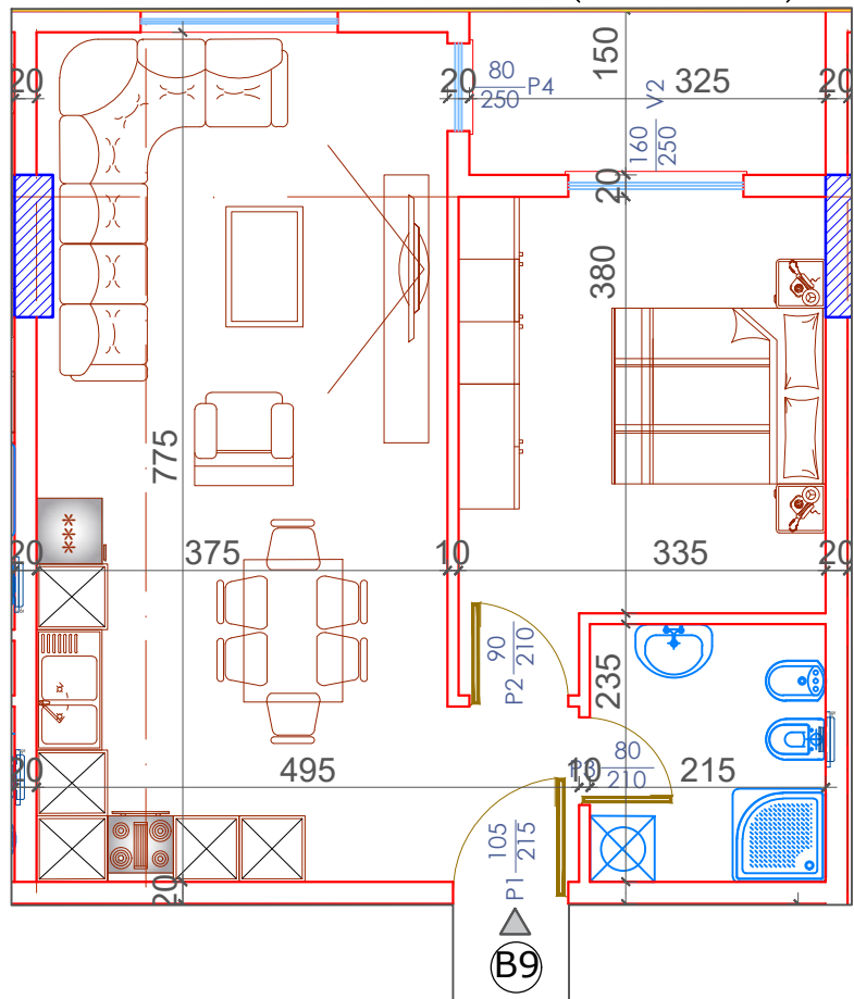
PLANIMETRIA E APARTAMENTIT NR 9 KATI TIP (KATI DYTË +8.19) SEKSIONI B SH.1:75
