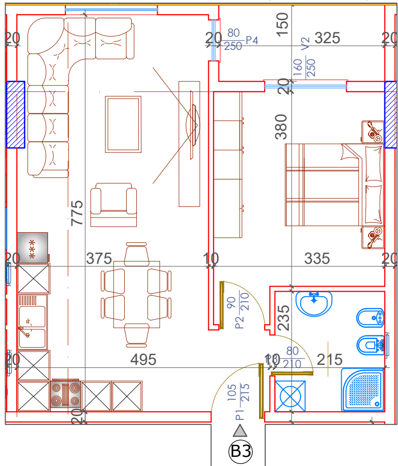
PLANIMETRIA E APARTAMENTIT NR 3 KATI TIP (KATI PARË +5.04) SEKSIONI B SH.1:100
