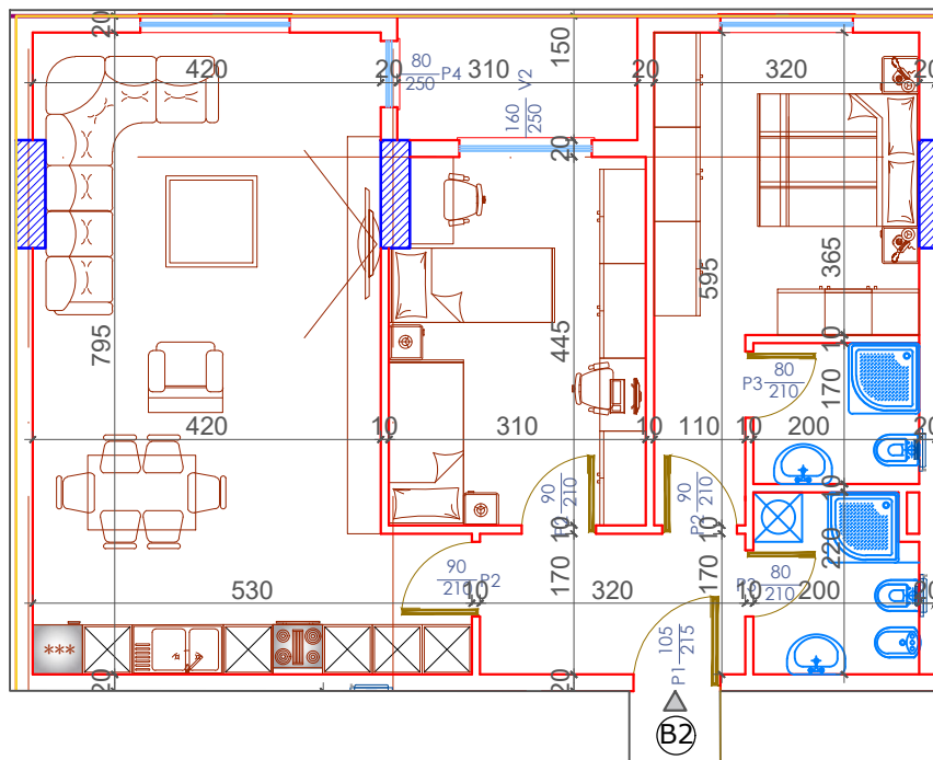
PLANIMETRIA E APARTAMENTIT NR 2 KATI TIP (KATI PARË +5.04) SEKSIONI B SH.1:100
