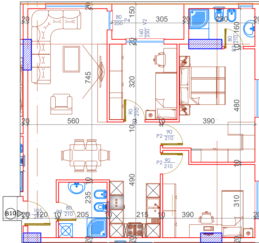
PLANIMETRIA E APARTAMENTIT NR 10 KATI TIP (KATI DYTË +8.19) SEKSIONI B
