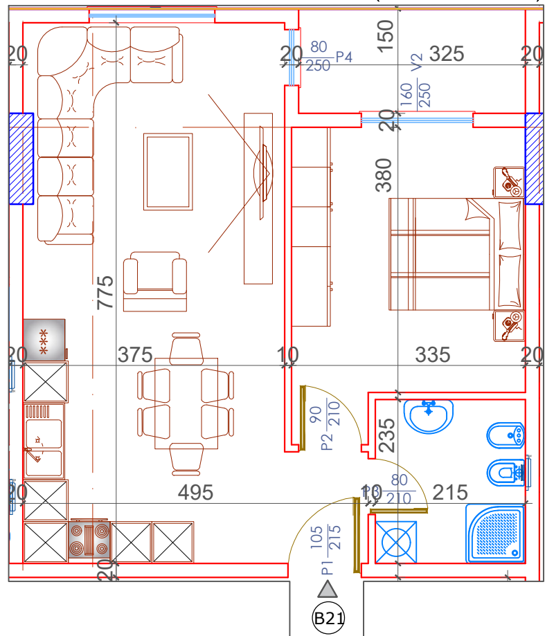
PLANIMETRIA E APARTAMENTIT NR 21 KATI TIP (KATI KATËRT +14.49) SEKSIONI B SH.1:75
