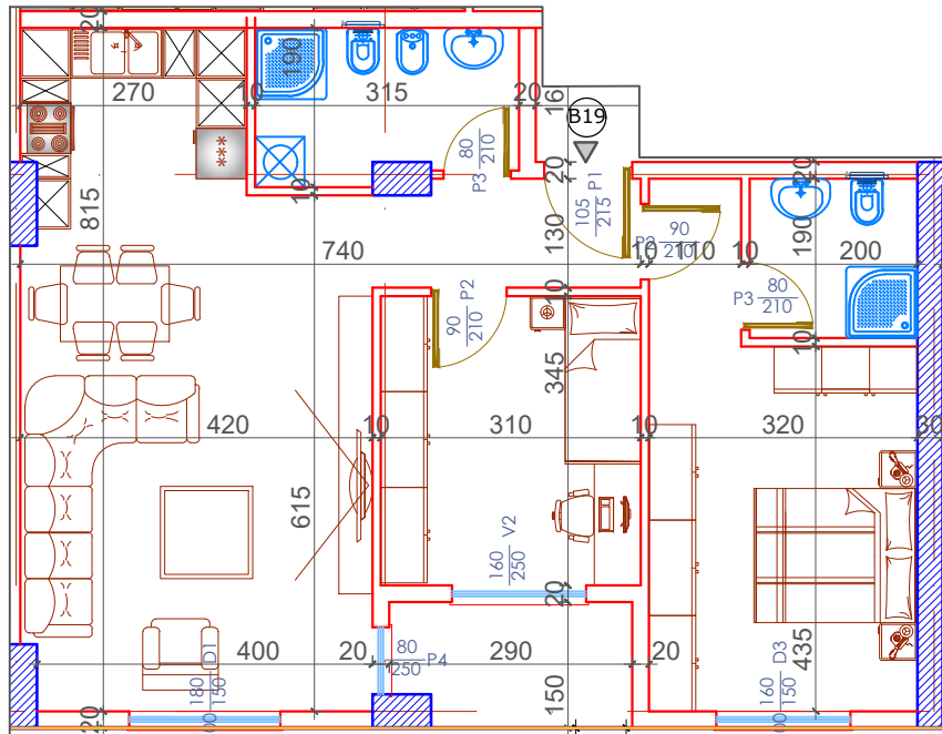
PLANIMETRIA E APARTAMENTIT NR 19 KATI TIP (KATI KATËRT +14.49) SEKSIONI B SH.1:100
