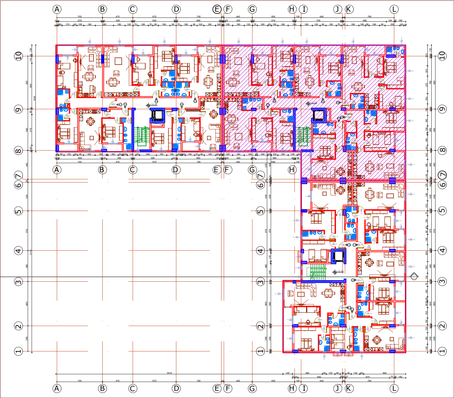
PLANIMETRIA E KATIT TIP (KATI KATËRT +14.49) , SEKSIONI A SH 1:350
