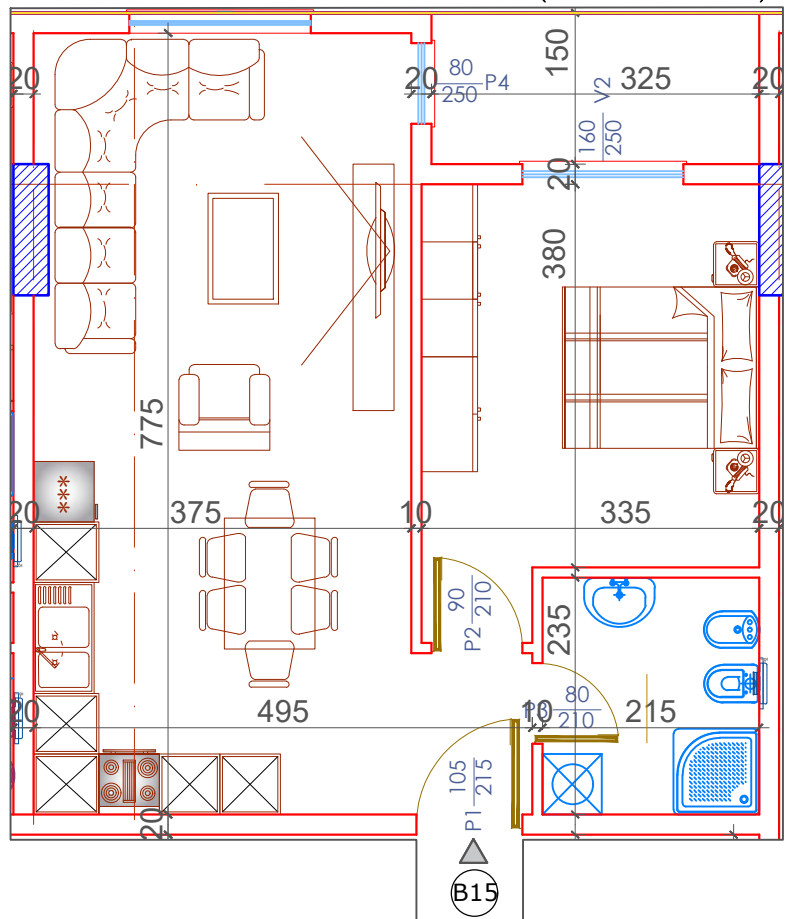
PLANIMETRIA E APARTAMENTIT NR 15 KATI TIP (KATI TRETË +11.34) SEKSIONI B SH.1:75
